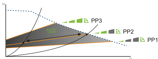
22. ábra Három arányos-nyomás görbe/beállítás
