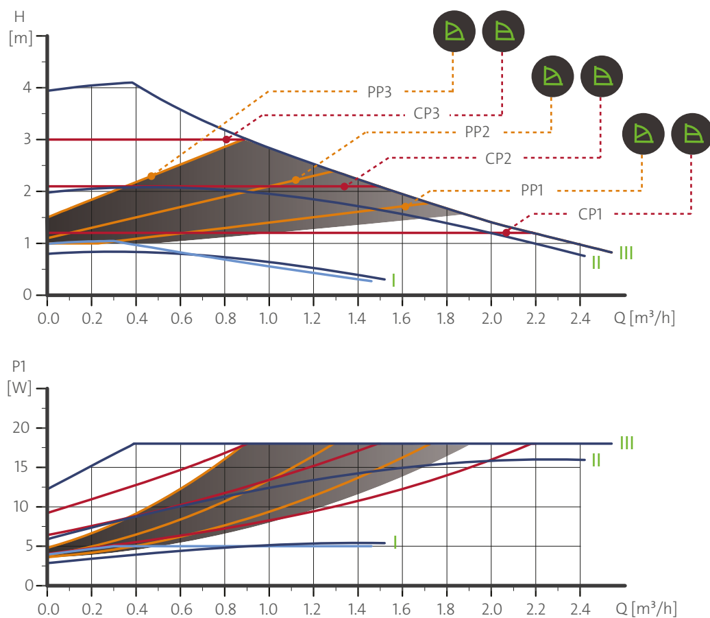
37. ábra ALPHA2 és ALPHA3, XX-40
