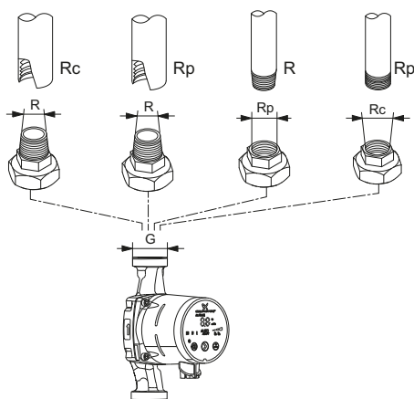
43. ábra G menetek és R menetek
