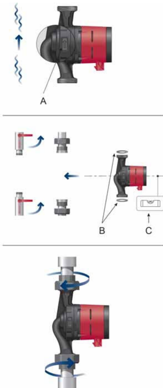
1. ábra Az ALPHA2 vagy az ALPHA3 telepítése
